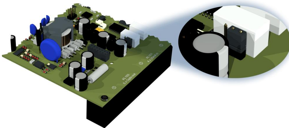
Puente de codificación 1 para configurar el contacto de relé 1 (X402/KL402)
