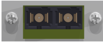
o cable de fibra óptica (SC-Duplex)
